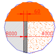
Détail B Echelle : 1/50
